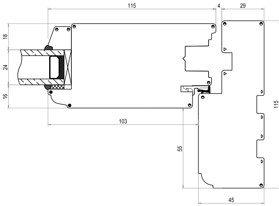
Tvårsnitt DOFAB KULTUR Utåtgående ytterdörr sidostycke ovanifrån
